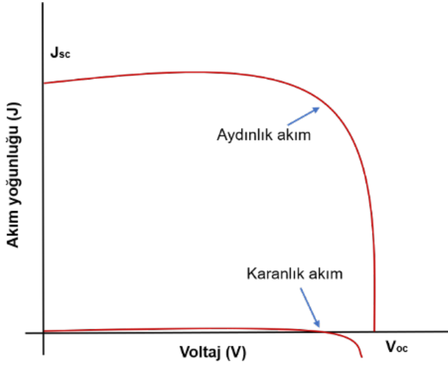
Şekil 2.19 Aydınlık ve karanlıkta ideal diyotun akım-gerilim karakteristiği.
