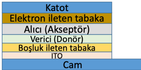
Şekil 2.12 Çift katmanlı (bilayer) güneş gözesi yapısı.
