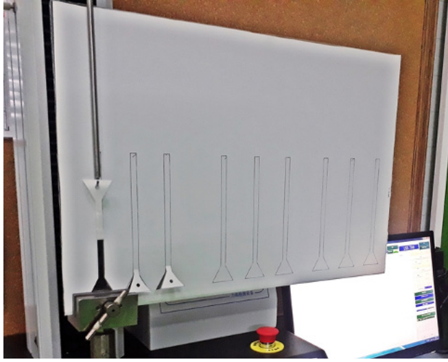
Şekil 3.5. Enkapsülant-Cam-Arka tabaka (Backsheet) Çekme (Peeling) Testi
