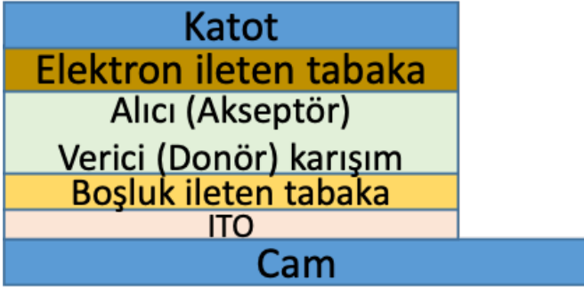
Şekil 2.13 Hacimli heteroeklem organik güneş gözesi yapısı.
