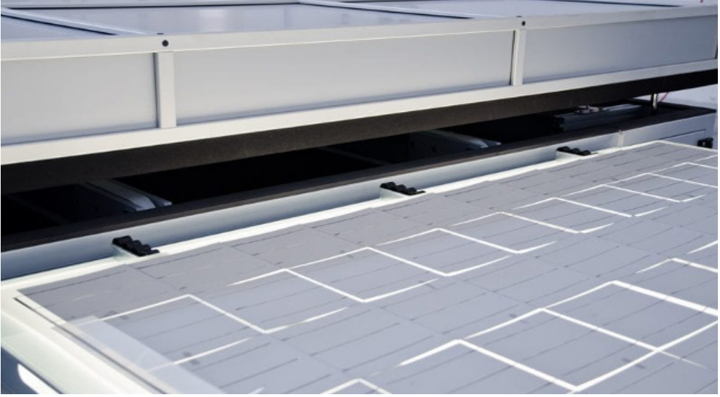
Şekil 3.8. Laminasyon öncesi Elektrolüminesans kontrol
