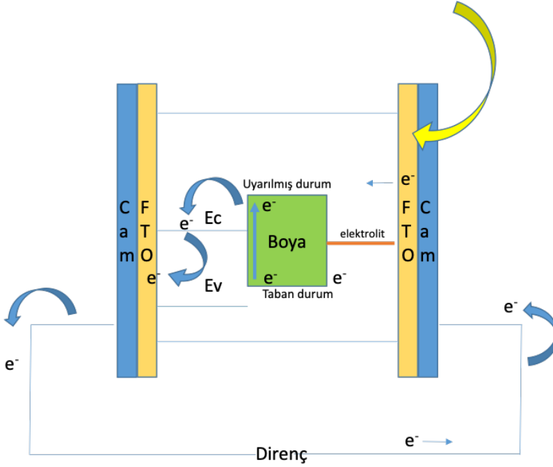
Şekil 2.10 Boya Bazlı Güneş Gözelleri çalışma prensibi
