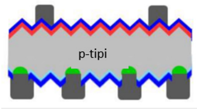
Şekil 2.5 İki yüzlü (Bifacial cell) göze tasarımı
