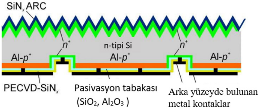
Şekil 2.6 Arka kontaklı arka eklemli güneş gözesi
