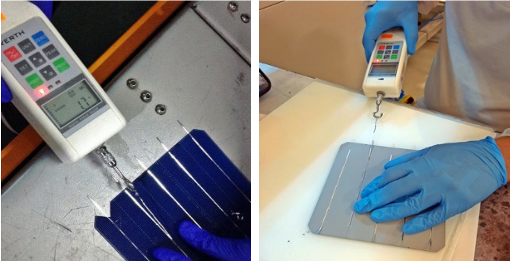
Şekil 3.4. Hücre-Ribbon Çekme (Peeling) Testi
