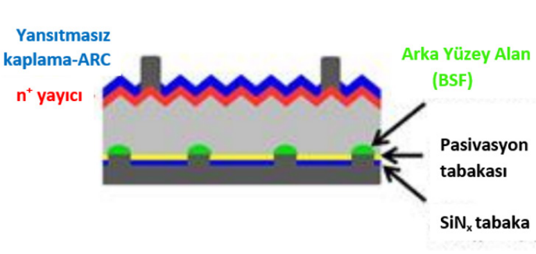
Şekil 2.4 Pasive edilmiş yayıcı arka kontak gözeler (Passivated Emitter Rear contact Cell-PERC)
