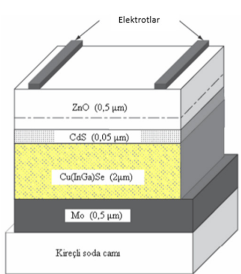
Şekil 2.9 Tipik bir \text{Cu(InGa)Se}_2 güneş gözesinin kesit görünümü
