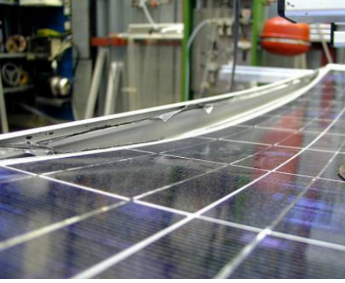
Şekil 3.1. Mekanik yük testi
